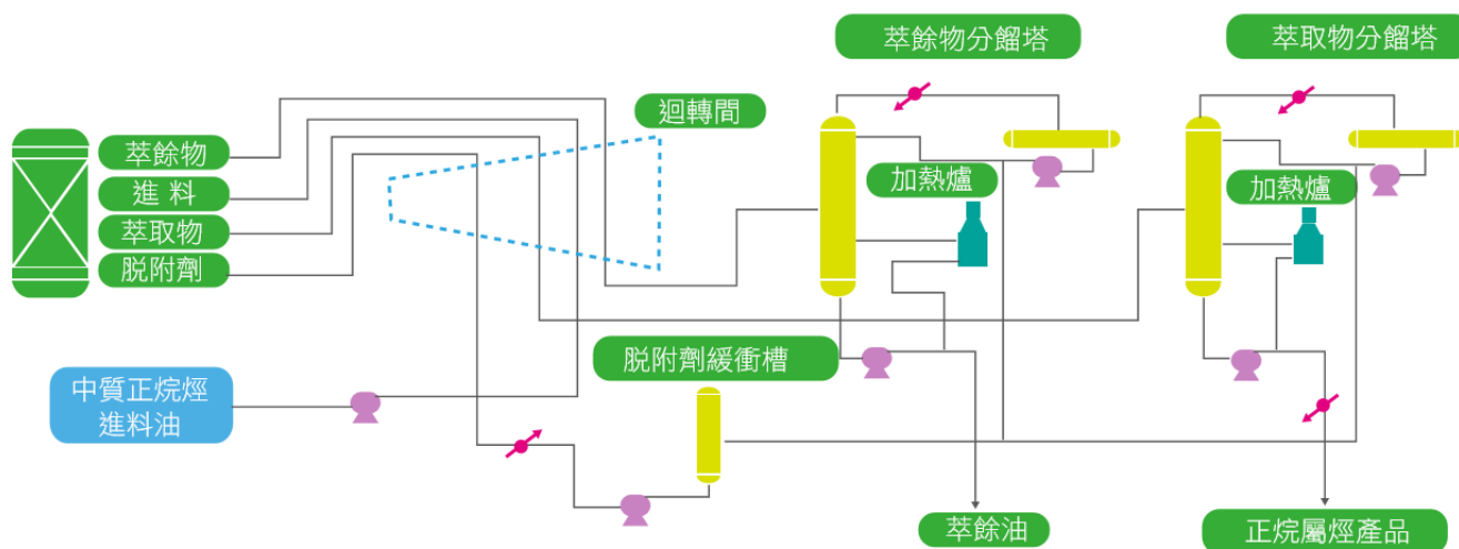
[ 正烷屬烴生產流程圖 ]
